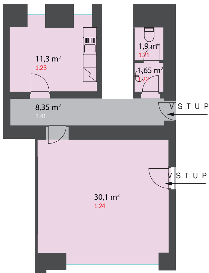
PŮDORYS PODLAŽÍ
