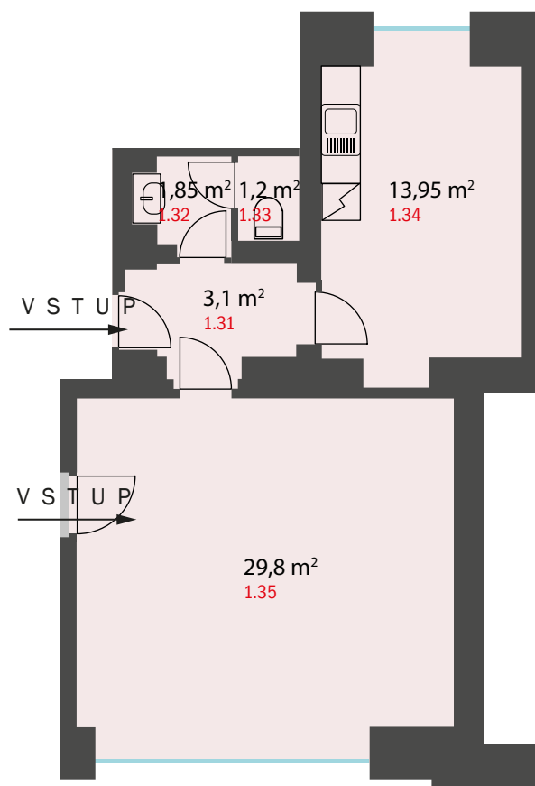
PŮDORYS PODLAŽÍ
