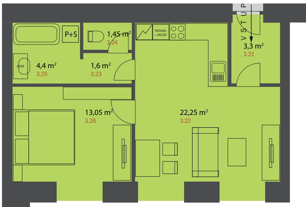
PŮDORYS PODLAŽÍ
