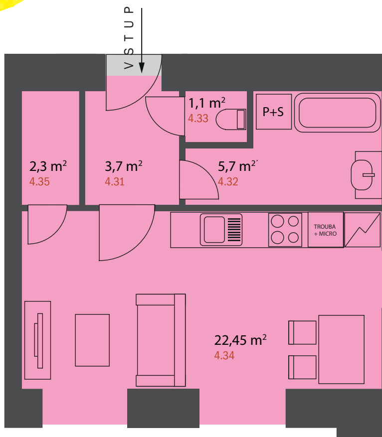
PŮDORYS PODLAŽÍ
